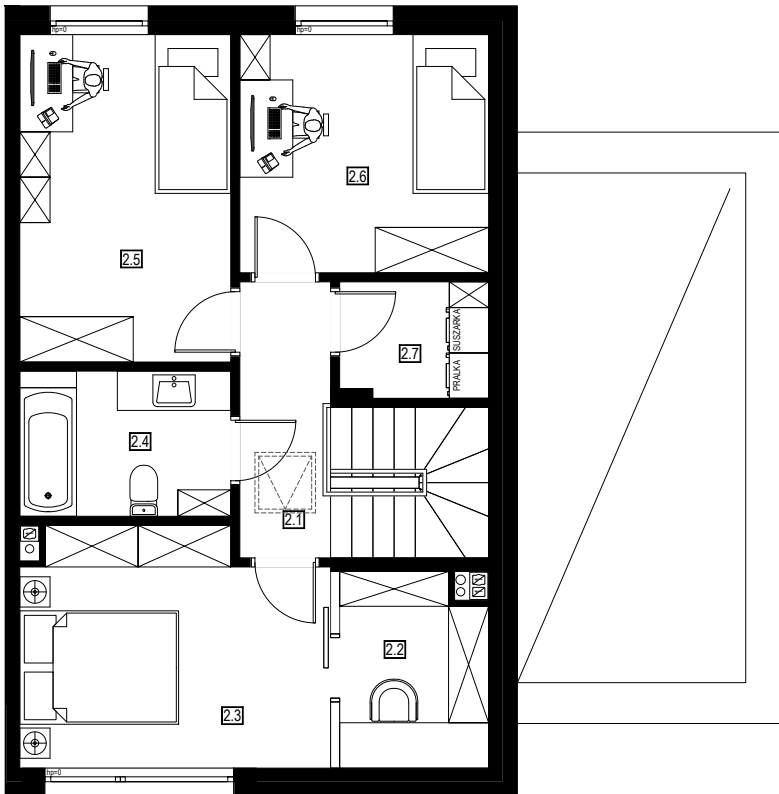
Rzut piętra
