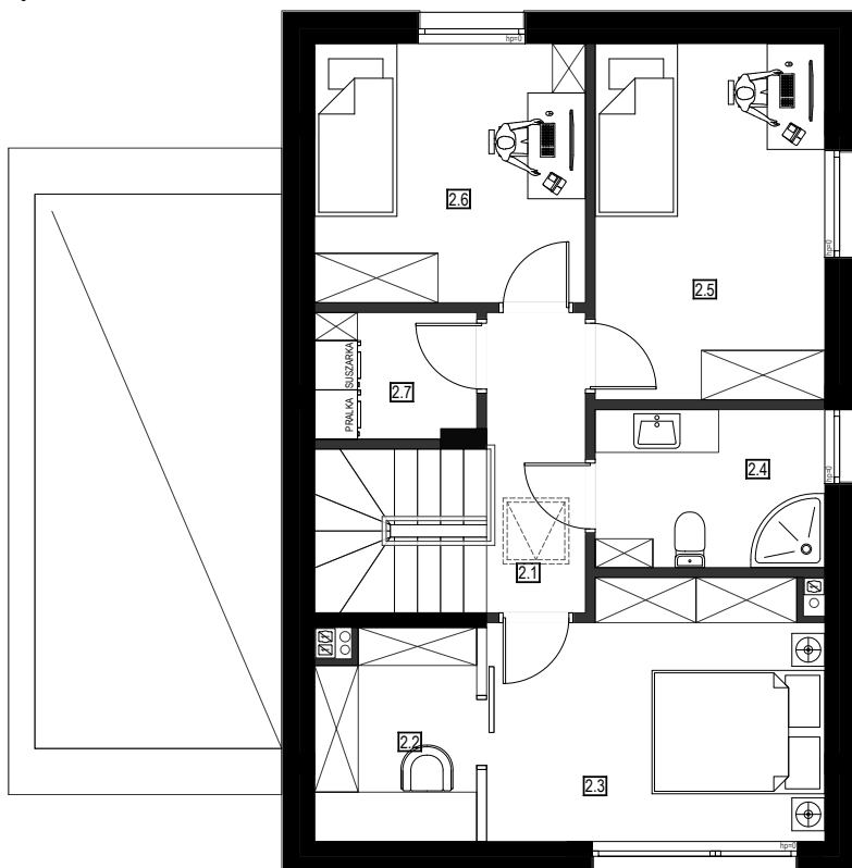
Rzut piętra
