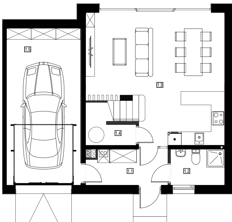
Rzut parteru
